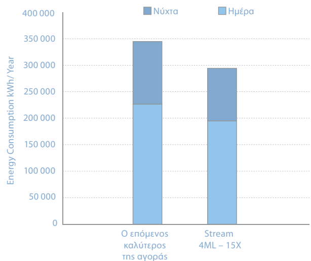
Σχέδιο 4: Σύγκριση μεταξύ Stream και του επόμενου καλύτερου της αγοράς.
