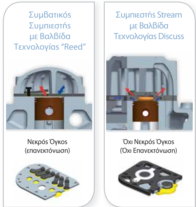
Σχέδιο 2. Η βασική διαφορά στην τεχνολογία Βαλβίδων μεταξύ συμβατικών και Stream συμπιεστή.
